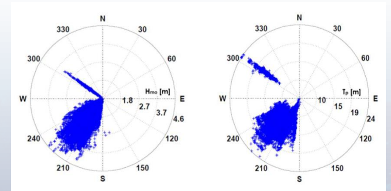
Rosas de Dispersión de Oleaje en aguas profundas
