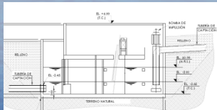
Cuarto de impulsión
