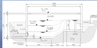
Cámara de carga
